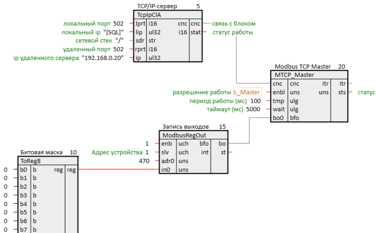
Рисунок 5.19 – Настройка обмена с модулем MK210-311
