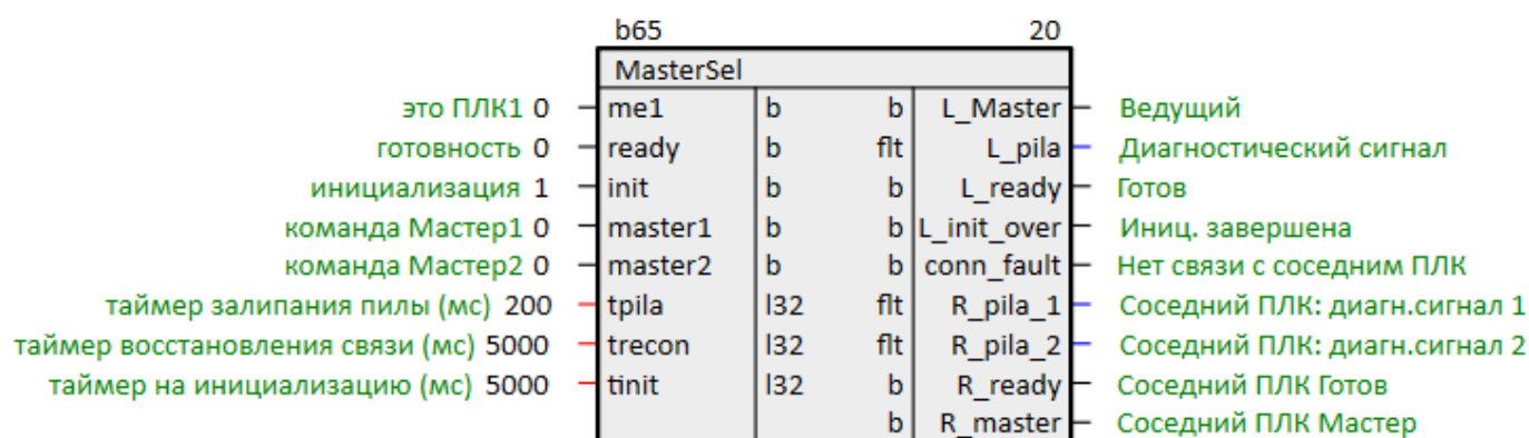
Рисунок 2.5 – Определение ведущего (MasterSel)
