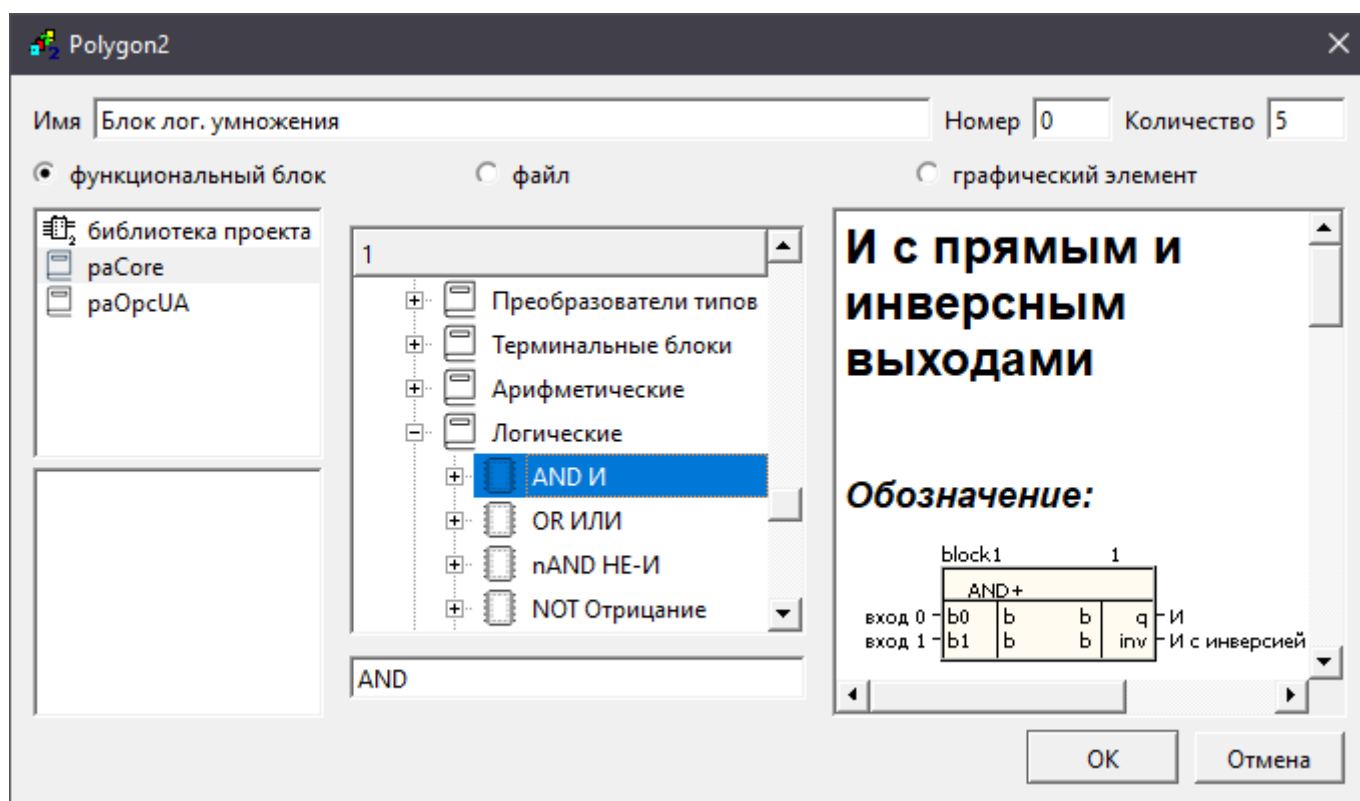
Рисунок 4.18 – Окно создания функционального блока
