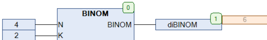
Рис. 5.16. Пример работы с функцией BINOM на языке CFC
