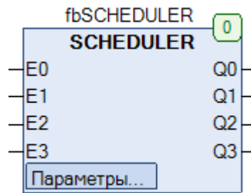
Рис. 15.24. Внешний вид ФБ SCHEDULER на языке CFC
