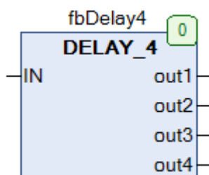
Рис. 19.13. Внешний вид ФБ DELAY_4 на языке CFC
