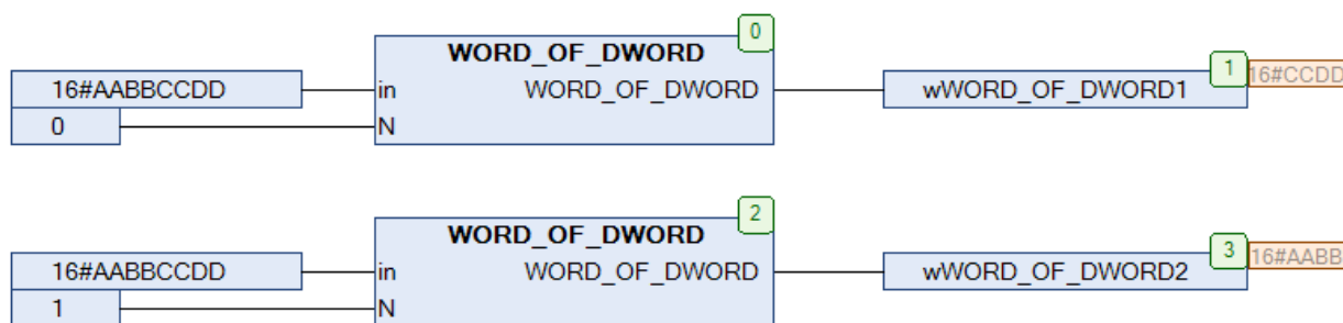
Рис. 16.81. Пример работы с функцией WORD_OF_DWORD на языке CFC
