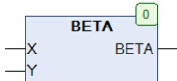
Рис. 5.13. Внешний вид функции БЕТА на языке CFC
