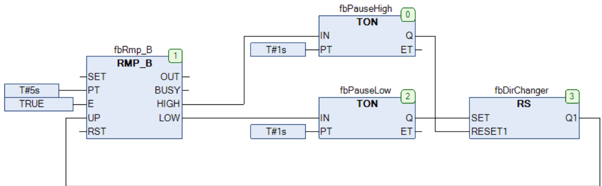
Рис. 18.27. Пример работы с ФБ RMP_B на языке CFC
