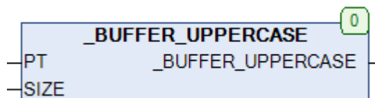
Рис. 25.8. Внешний вид функции _BUFFER_UPPERCASE на языке CFC
