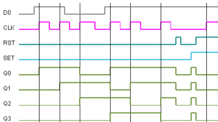
Рис. 17.15. Трассировка работы ФБ SHR_4E
