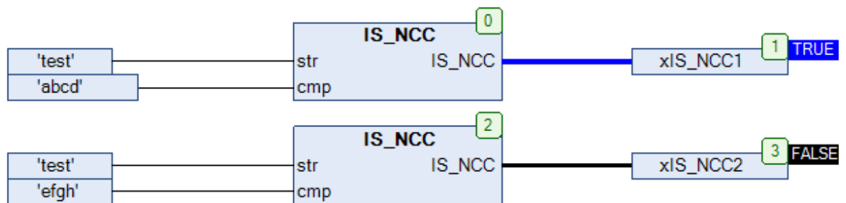
Рис. 13.92. Пример работы с функцией IS_NCC на языке CFC
