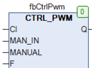
Рис. 23.13 Внешний вид ФБ CTRL_PWM на языке CFC
