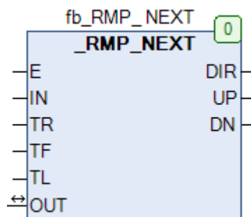
Рис. 18.3. Внешний вид ФБ _RMP_NEXT на языке CFC
