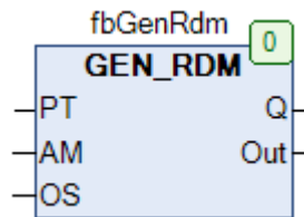
Рис. 18.10. Внешний вид ФБ GEN_RDM на языке CFC
