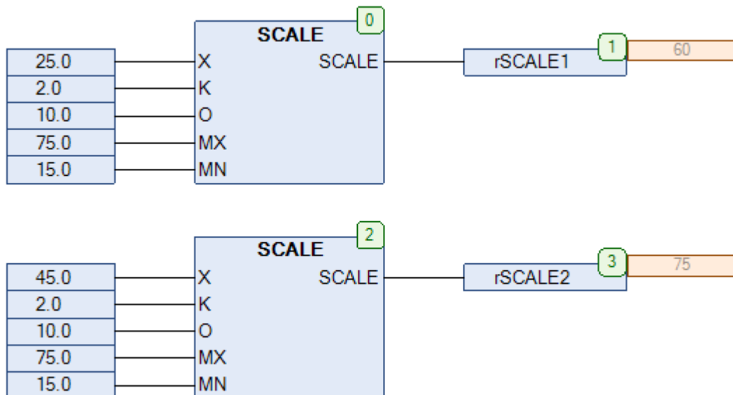
Рис. 19.45. Пример работы с функцией SCALE на языке CFC
