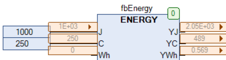
Рис. 22.17. Внешний вид ФБ ENERGY на языке CFC (конвертация суммы значений)
