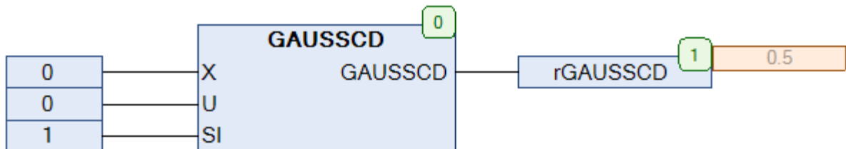
Рис. 5.64. Пример работы с функцией GAUSSCD на языке CFC
