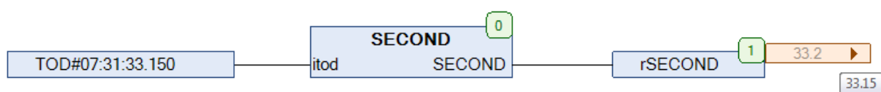
Рис. 12.83. Пример работы с функцией SECOND на языке CFC
