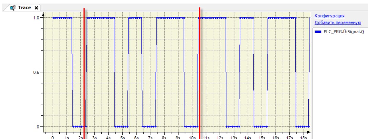
Рис. 24.21. Трассировка ФБ SIGNAL
