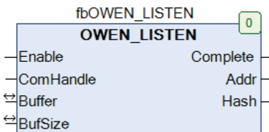
Рис. 3.12. Внешний вид ФБ OWEN_LISTEN на языке CFC
