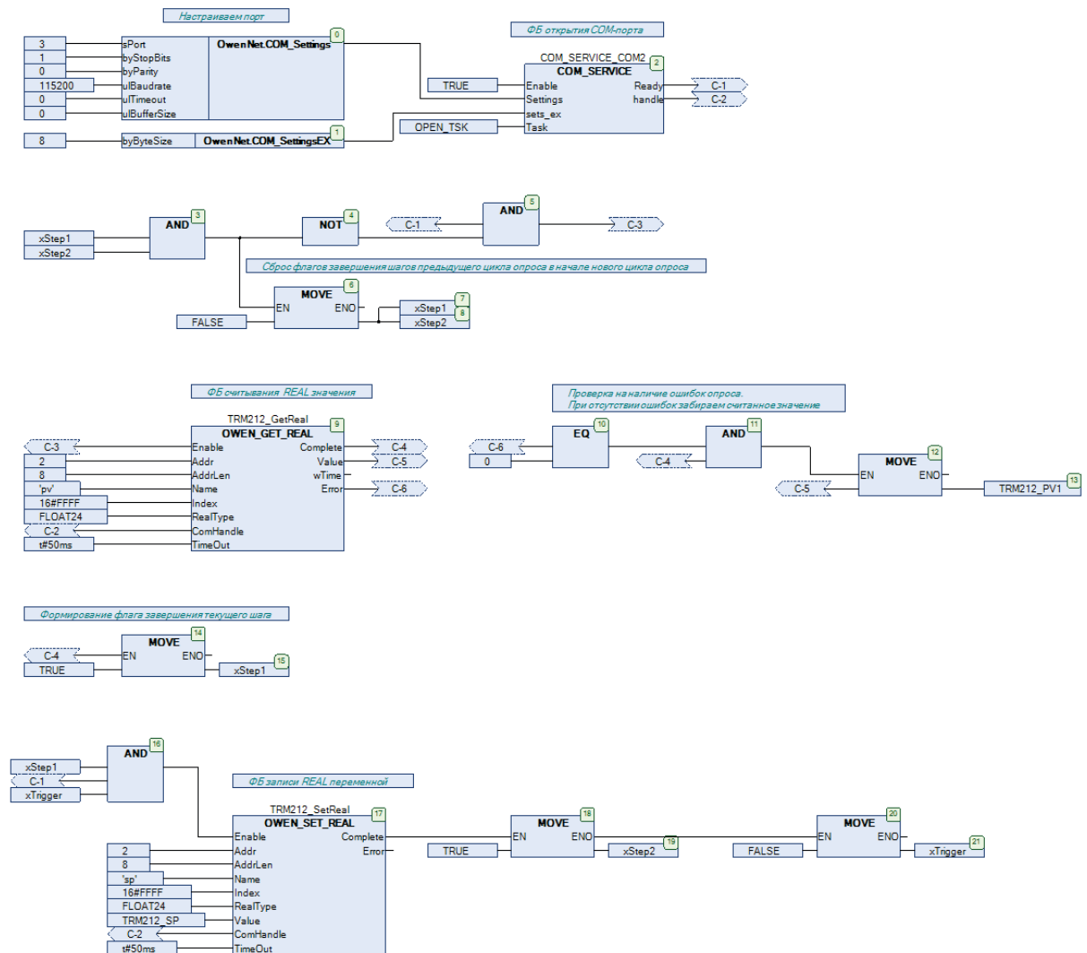
Рис. 4.3. Код программы PLC_PRG (CFC)
