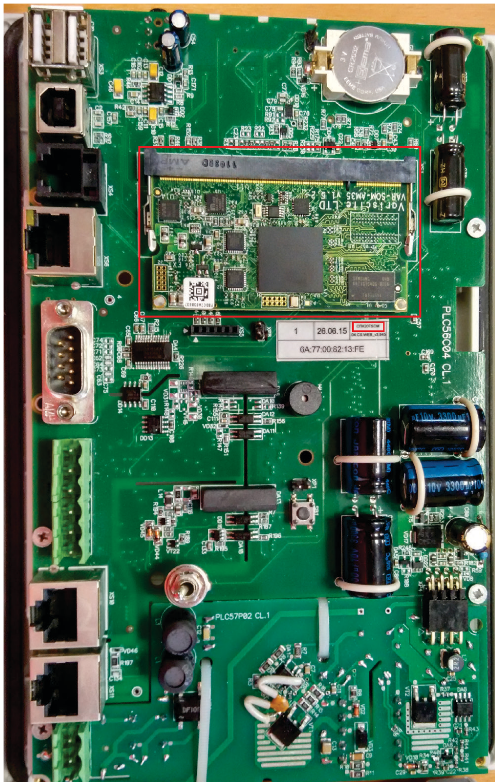
Рис. 6.5. Внешний вид платы M02
