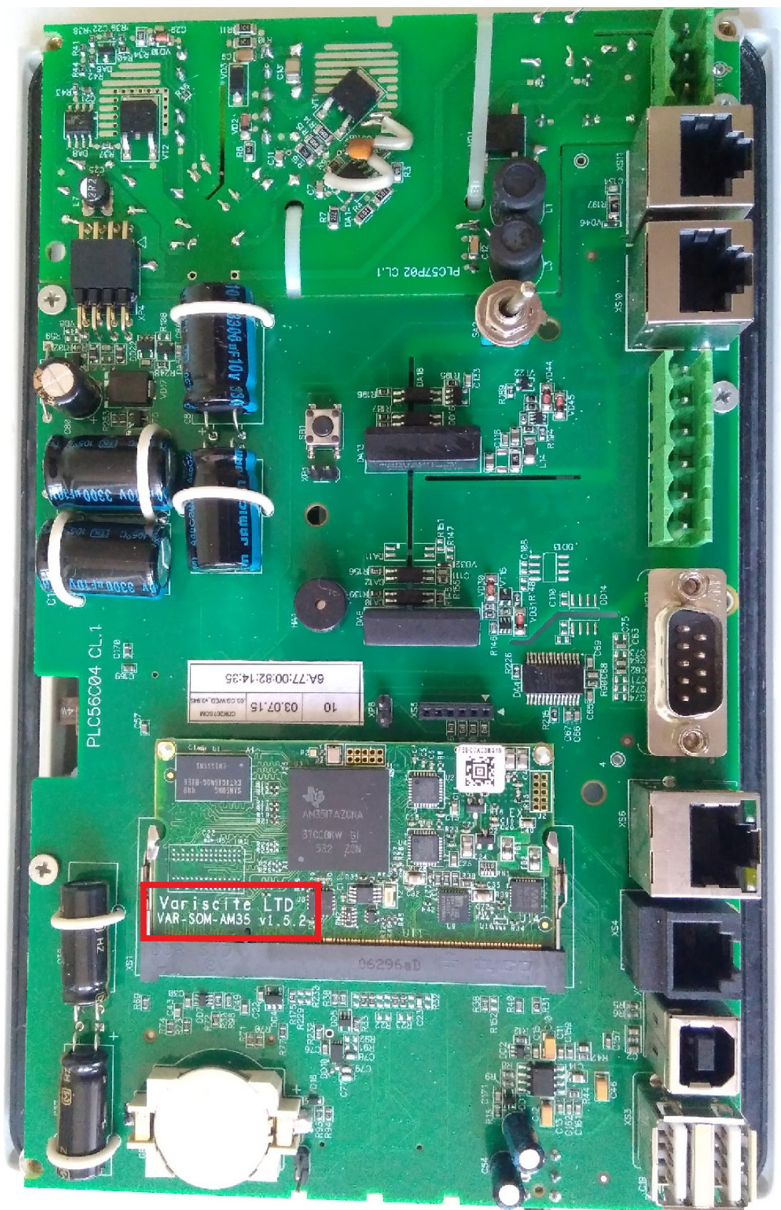
Рис. 6.5. Внешний вид платы M02
