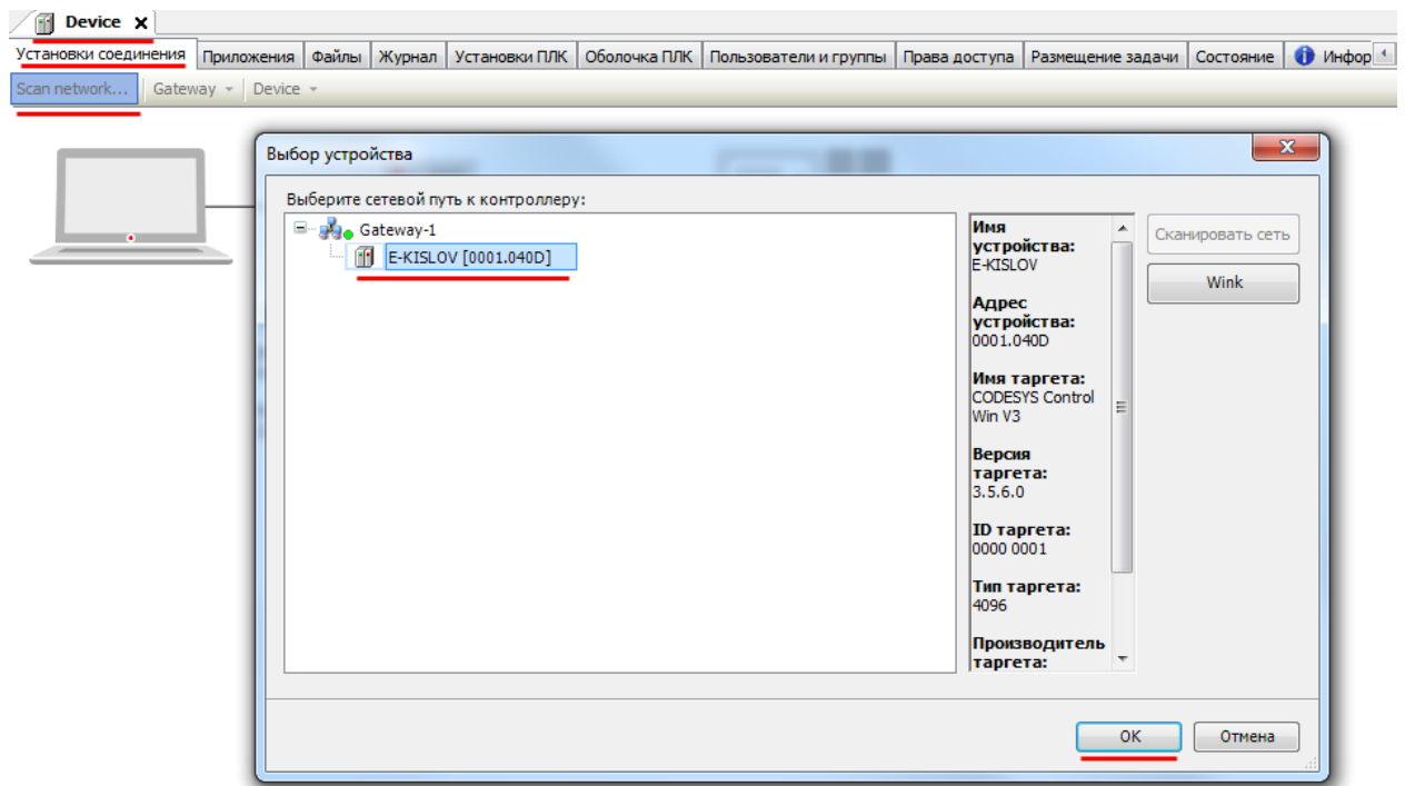
Рис. 7.29. Установка связи с виртуальным контроллером
