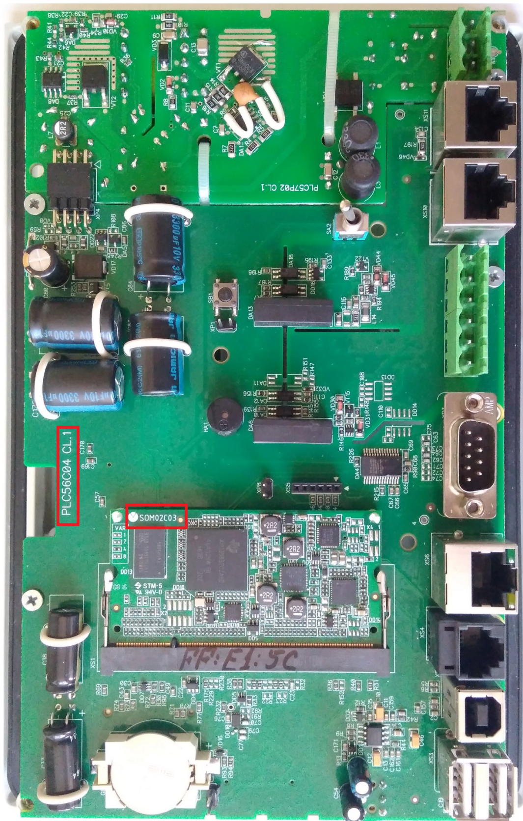
Рис. 6.6. Внешний вид платы M04
