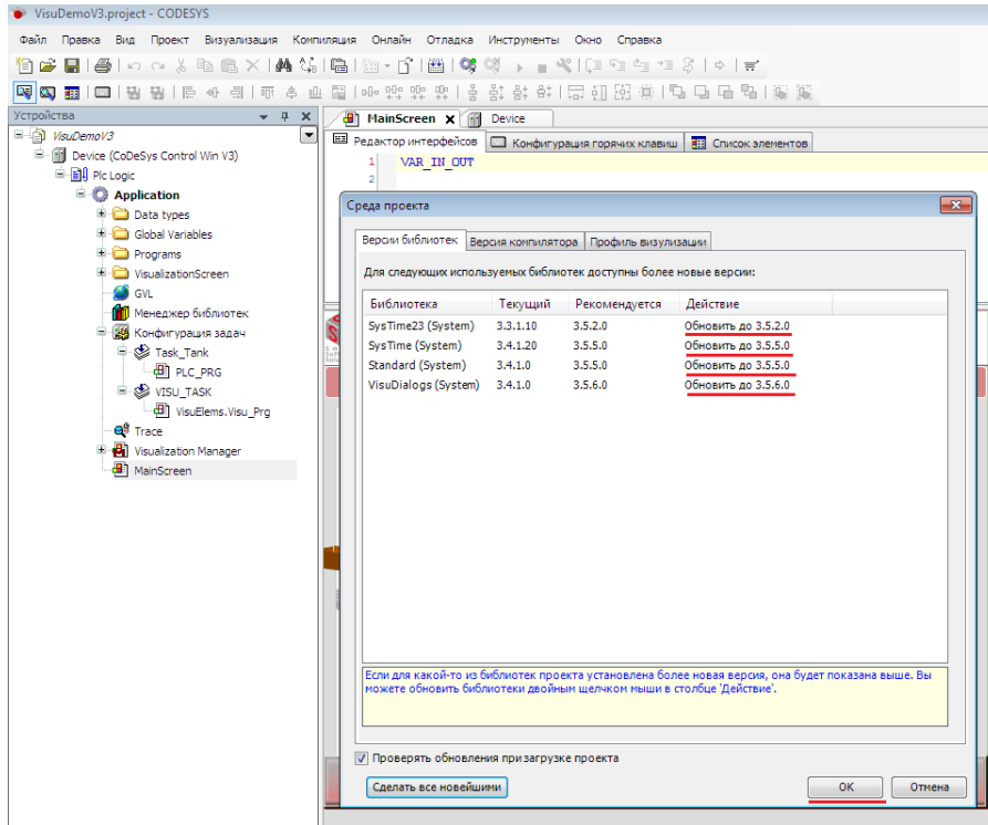
Рис. 7.36. Обновление компонентов проекта
