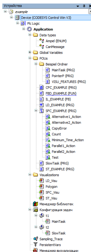
Рис. 7.13. Панель устройств CODESYS V3.5 SP6 (проект example)
